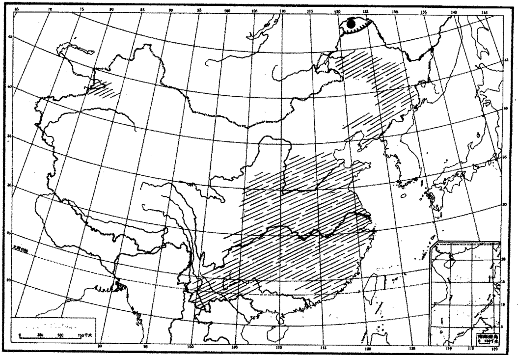
图 26 燕雀 Fringilla montifringilla 分布图
