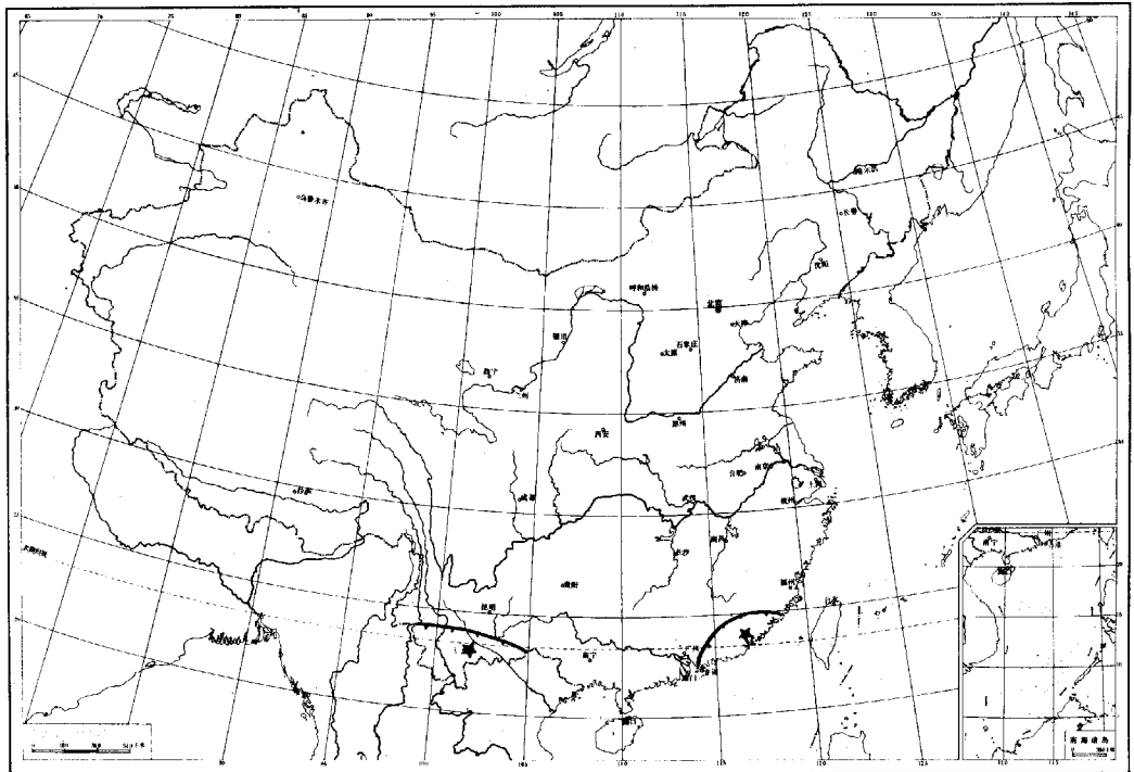
图68 金冠树八哥 Ampeliceps coronatus 的分布图
