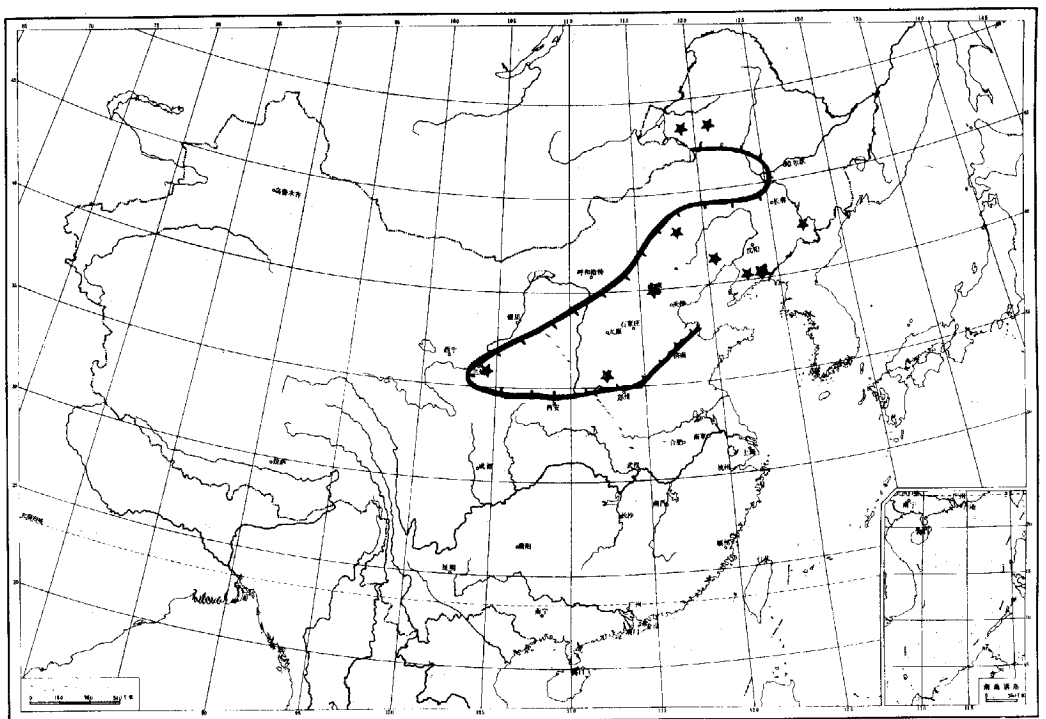
图49 北椋鸟 Sturnus sturninus 的分布图
