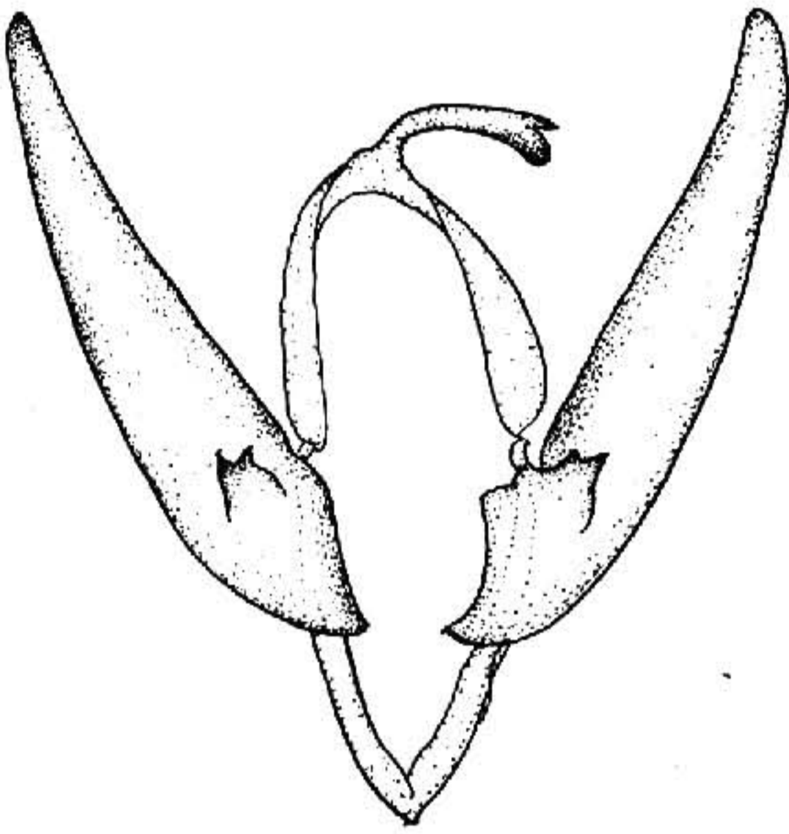
图 459 长斑幻夜蛾 Sasunaga longiplaga Warren ♂ 外生殖器
