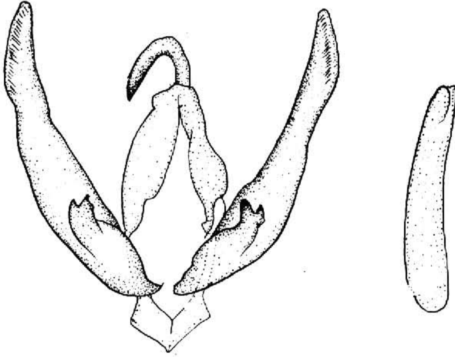
图 458 幻夜蛾 Sasunaga tenebrosa (Moore) ♂ 外生殖器
