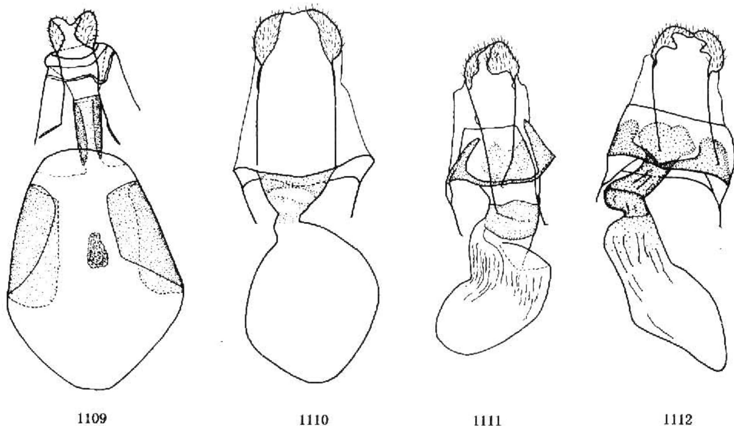
图 1109—1112 雌性外生殖器. 1109. 小周尺蛾 Perizoma parvaria (Leech); 1110. 愚周尺蛾 P. fatuaria (Leech); 1111. 白带周尺蛾 P. albofasciata (Moore); 1112. 对点周尺蛾 P. antisticta (Prout)
