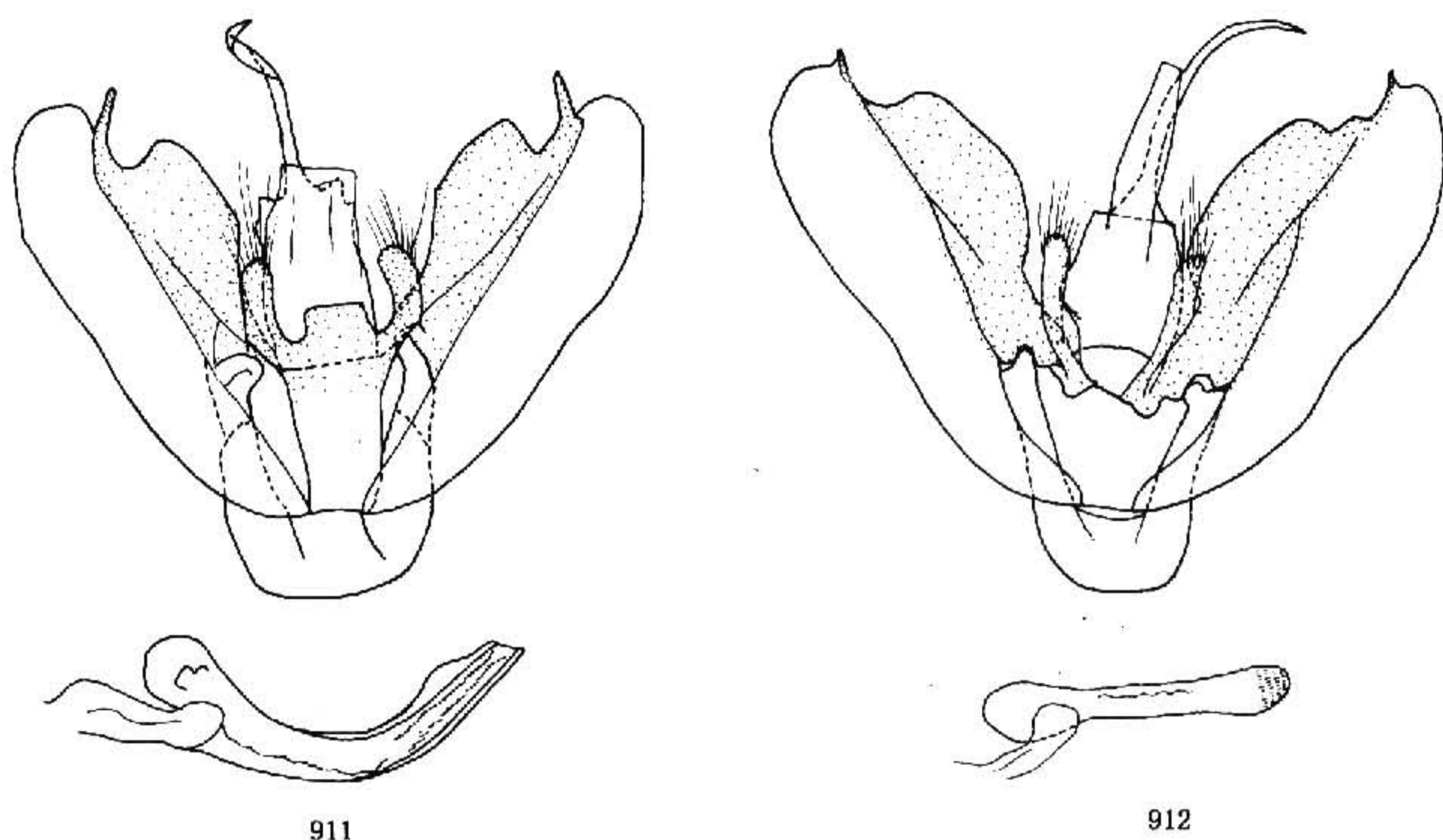
图 911—912 雄性外生殖器. 911. 哀羽带尺蛾 Pennithera lugubris Inoue (Inoue 玻片 12771 号); 912. 疏羽带尺蛾 P. manifesta Inoue (Inoue 玻片 13006 号)
