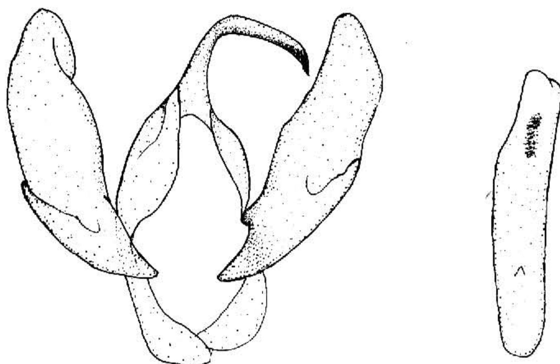
图 691 双点奴夜蛾 Paracolax bipuncta Owada ♂ 外生殖器
