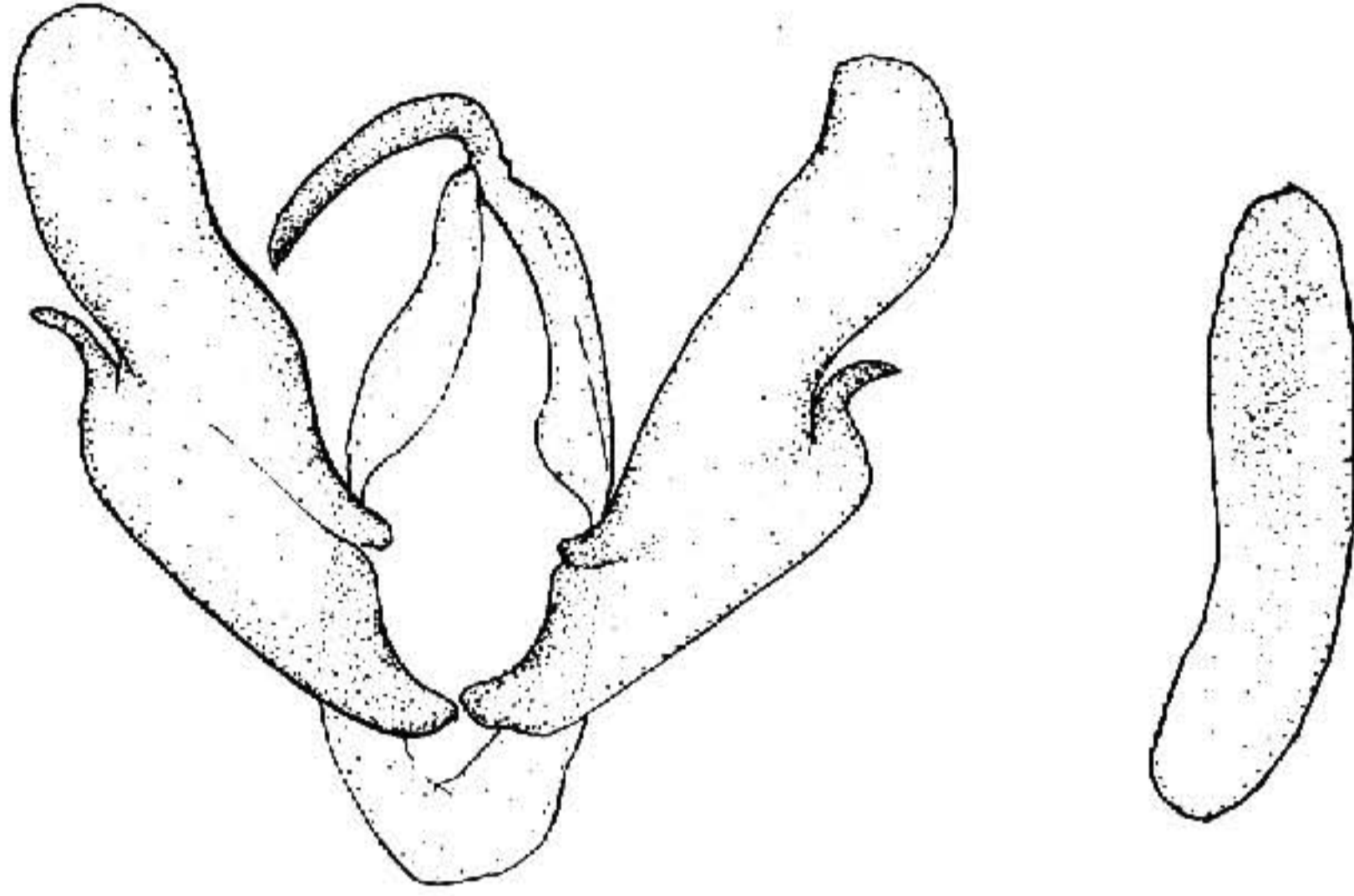
图 689 乐奴夜蛾 Paracolax angulata (Wileman) ♂ 外生殖器
