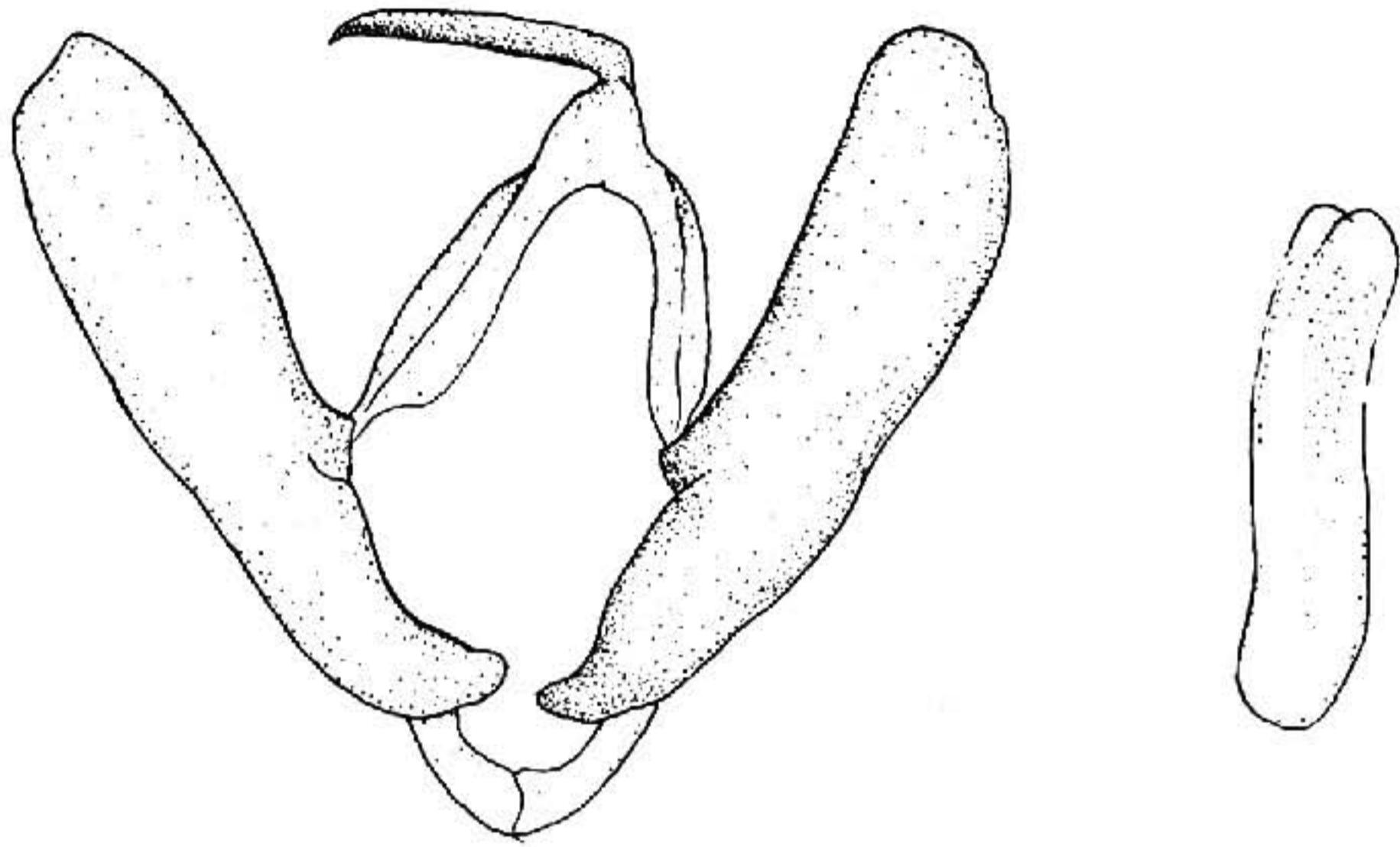
图 690 黄肾奴夜蛾 Paracolax pryeri (Butler) ♂ 外生殖器
