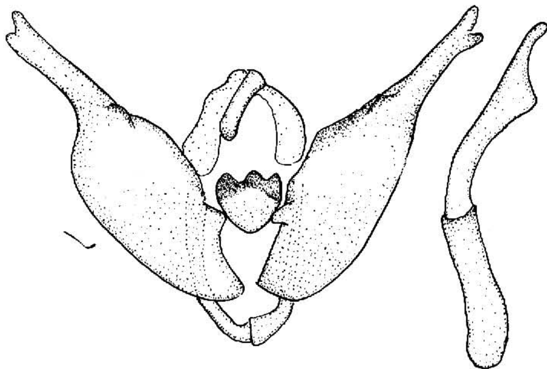
图 305 冥夜蛾 Erebophasma haematina Boursin ♂ 外生殖器
