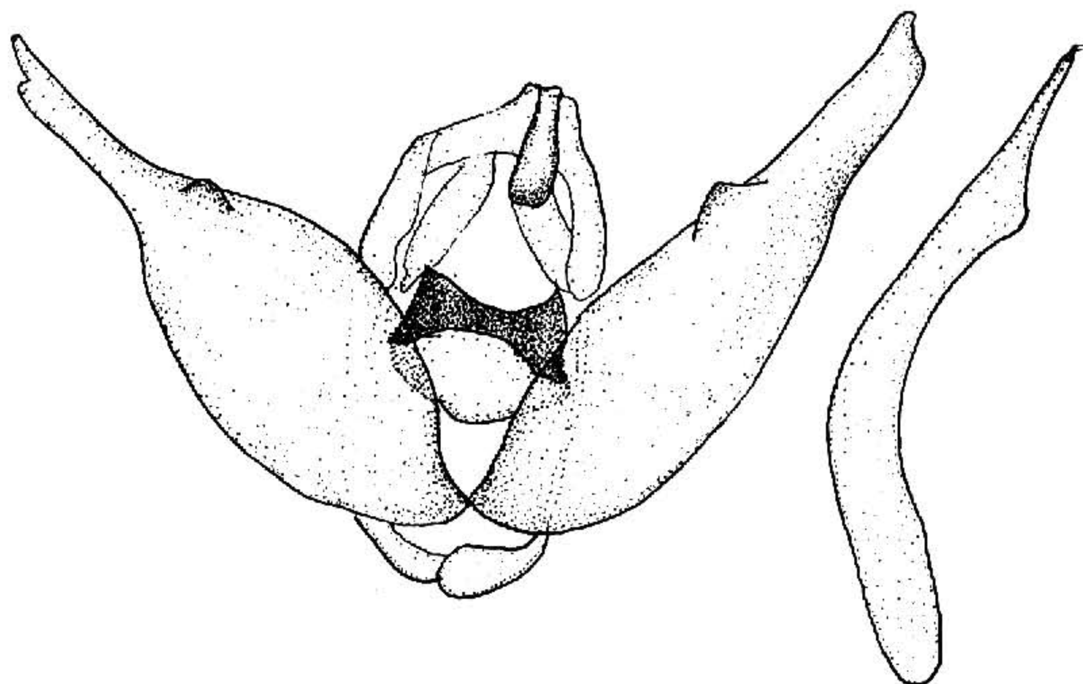
图 304 连纹冥夜蛾 Erebophasma conjunctiva Chen ♂ 外生殖器
