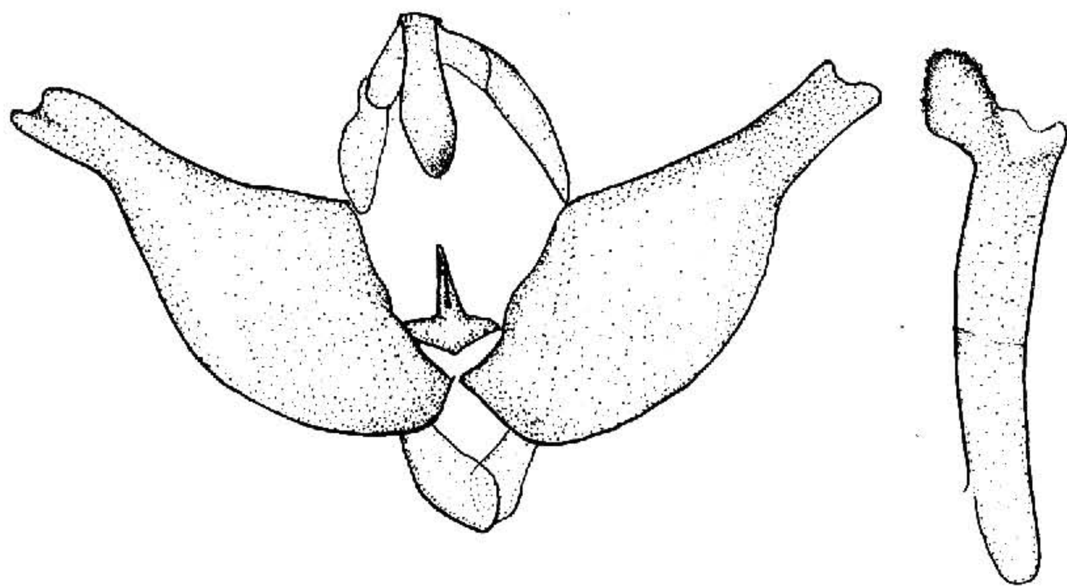
图 303 会冥夜蛾 Erebophasma vittata (Staudinger) ♂ 外生殖器
