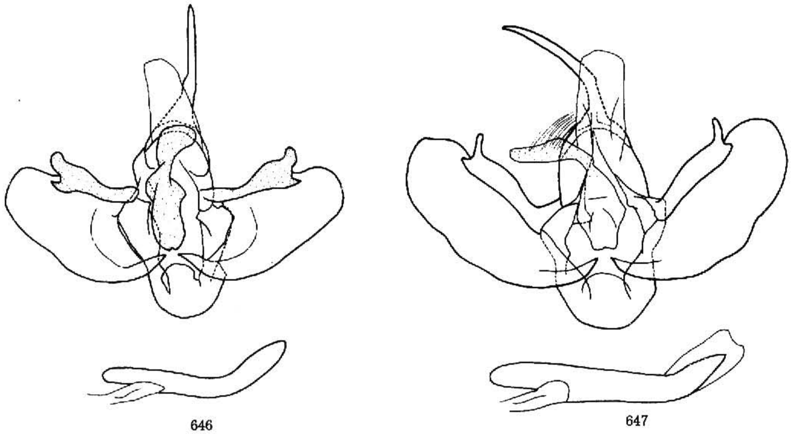
图 646—647 雄性外生殖器. 646. 间石尺蛾 Entephria intermediaria (Alphéraky); 647. 西藏灰石尺蛾 E. poliotaria tibetaria Aubert
