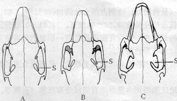
图2 云南兔三个亚种的头骨特征比较
