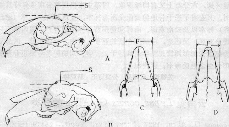
图1 云南兔和高原兔头骨特征比较
